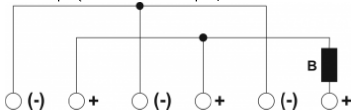
Schemat połączeń PIP-2AN z bezp. 0,375A
