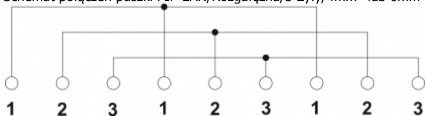
Schemat połączeń puszki PIP-2AN/Rozgałęźna/3 Żyły/4mm 2 lub 6mm 2
